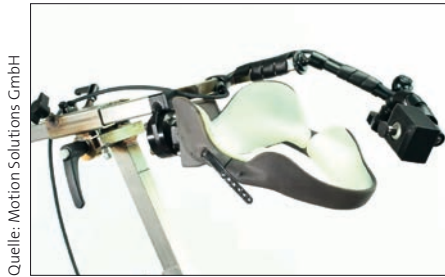
Bild 2: Die Bedienung erfolgt über eine Kopf-Zieh-Stütze, an die eine Kinnsteuerung angebaut ist
